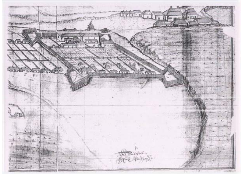
Егошихинский медеплавильный завод. Фрагмент плана, составленного М. Кутузовым. [1727–1729 гг.] ГАПК. Ф. р-2091. Оп. 1. Д. 45. Л. 4.
